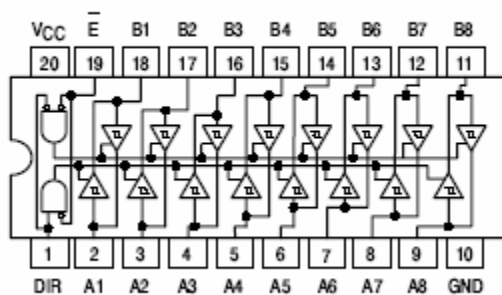
รูปที่ 3.4 โครงสร้างภายในของ HD74LS245P
