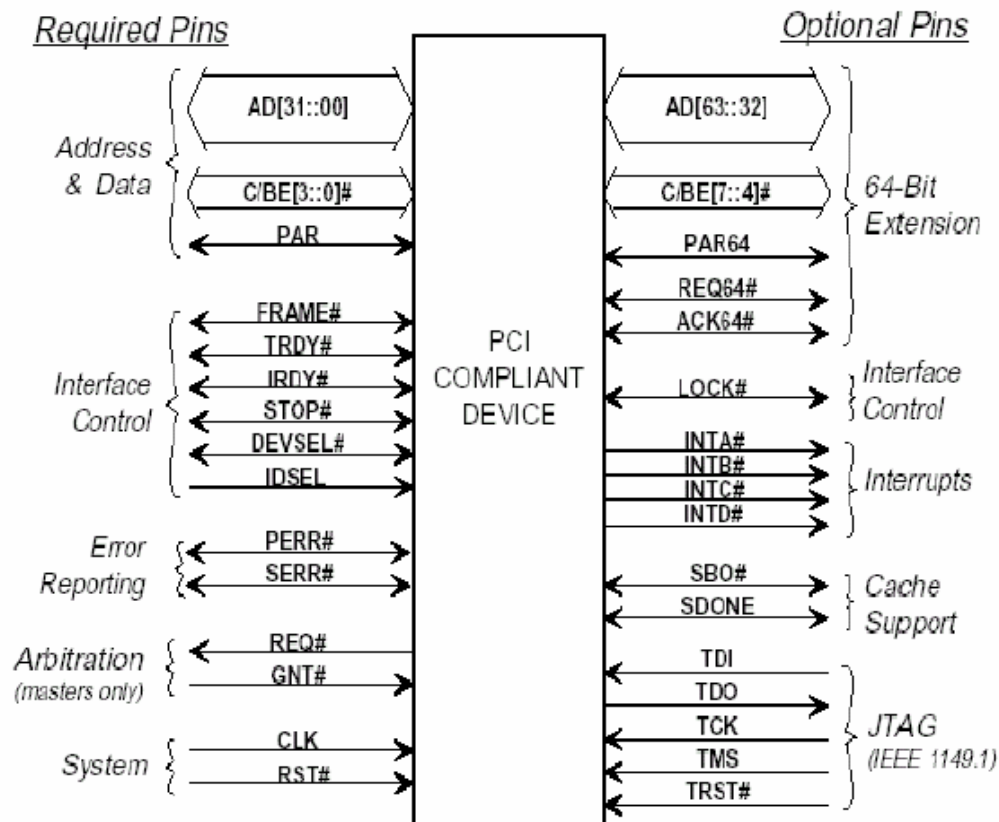
รูปที่ 3.6 สัญญาณอินเตอร์เฟสของ PCI BUS
