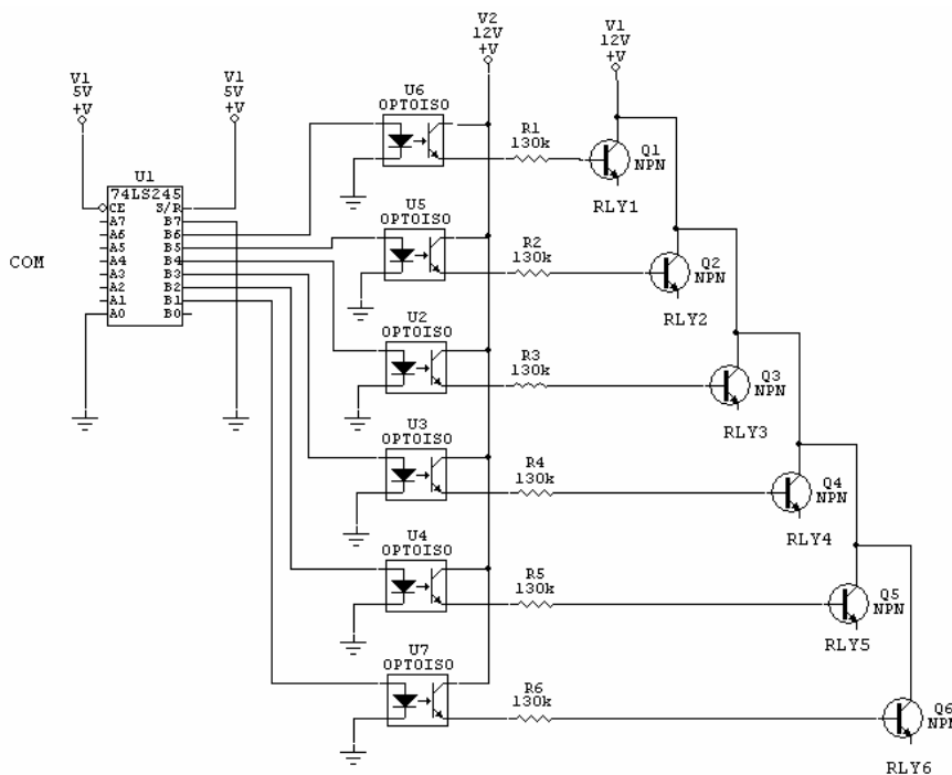
รูปที่ 3.5 วงจรของอุปกรณ์ปรับแรงดันไฟฟ้า
