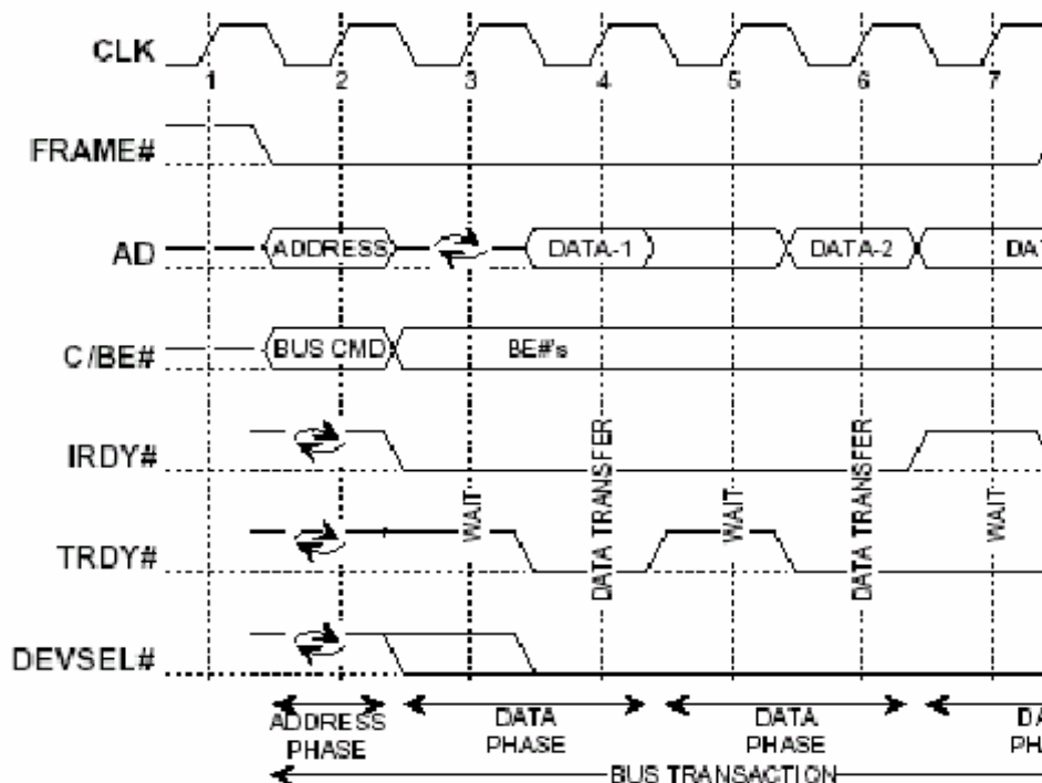
รูปที่ 3.7 Basic Read &amp; Write Operation
